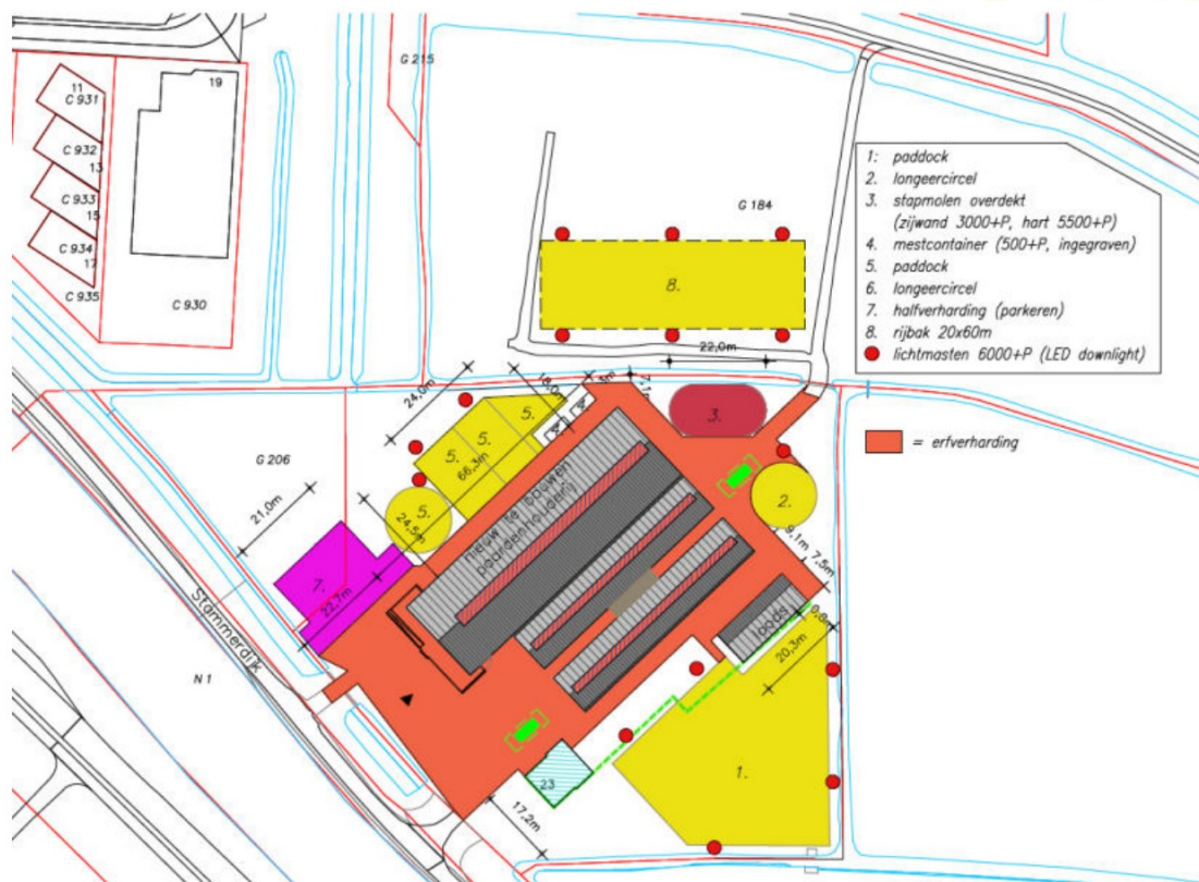
Figuur 4: Concept situatietekening van de nieuwe inrichting van het plangebied. Bron: DLV Advies.
